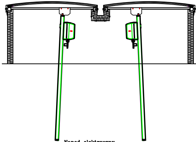
Napęd elektryczny D+H ZA 155/xxxx-BSY+HS SET
