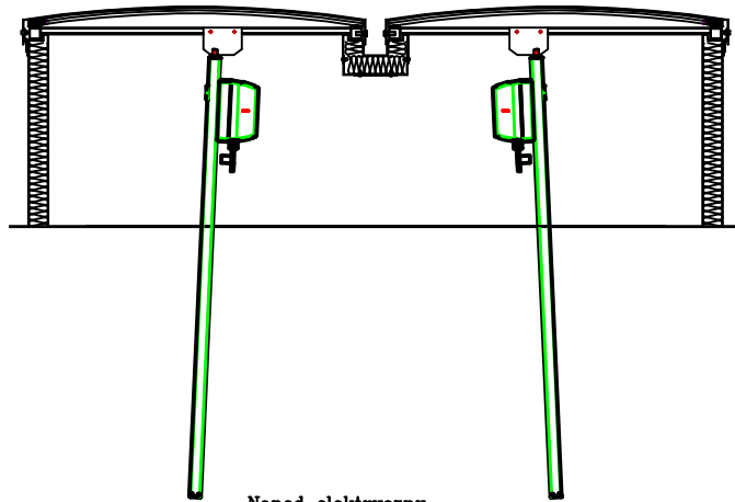
Naped elektryczny D+H ZA 155/xxxx-BSY+HS SET
