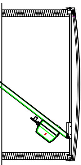
Naped elektryczny D+H ZA 156/xxxx-BSY+HS SET
